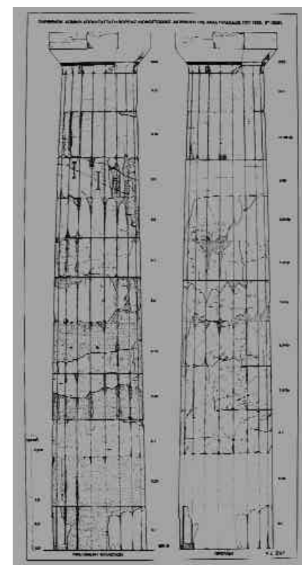
Πρόταση αποκατάστασης (δεξιά) 8ου (από Α.) Β. κίονα Παρθενώνος. Μελέτη Κ. Ζάμπα, 1998
