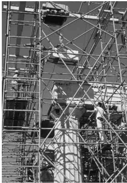
Εργασίες αποκατάστασης του Ν. τοίχου της Α. στοάς Προπυλαίων. Φωτ. Τ. Τανούλας, 2000
